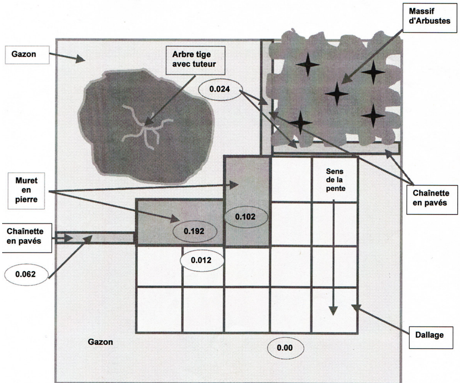
Plan échelle 1/20 ème
